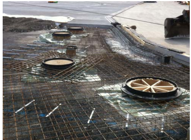
Plattenbewehrung inkl. Dilatationsfuge
